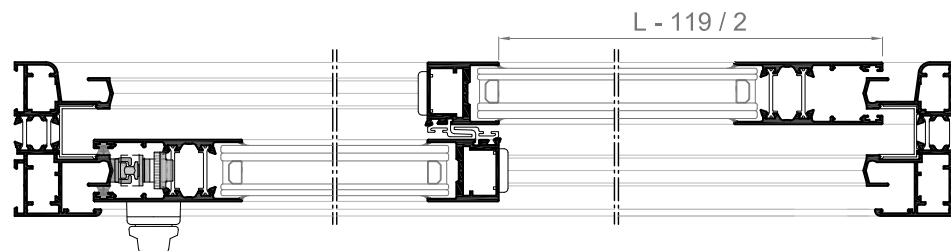
Sección A-A' / Hoja Minimalista
