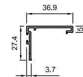
16704 Acople para hoja recta (16587M) Cruce 4135
