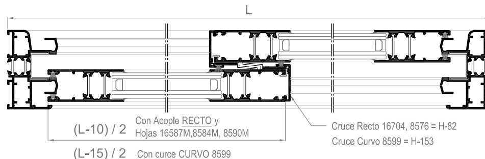
Sección A-A'
